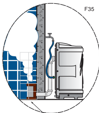
PREVER GRADE OU PROTEÇÃO DE SAÍDA DE VAPOR
