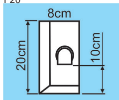
ALOJAMENTO DA SAÍDA DE VAPOR
