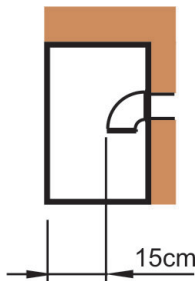
ALOJAMENTO DA SAÍDA DE VAPOR
